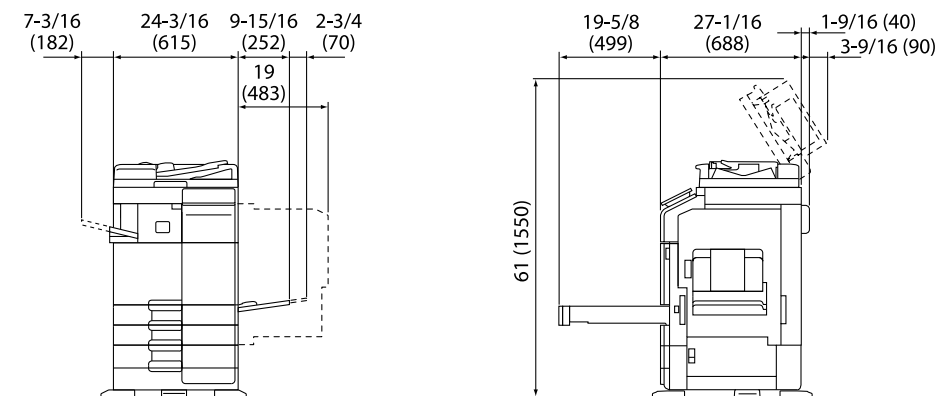
Βασική μονάδα + DF-632 + FS-533 + PC-216 Μονάδα: ίντσα (mm)
