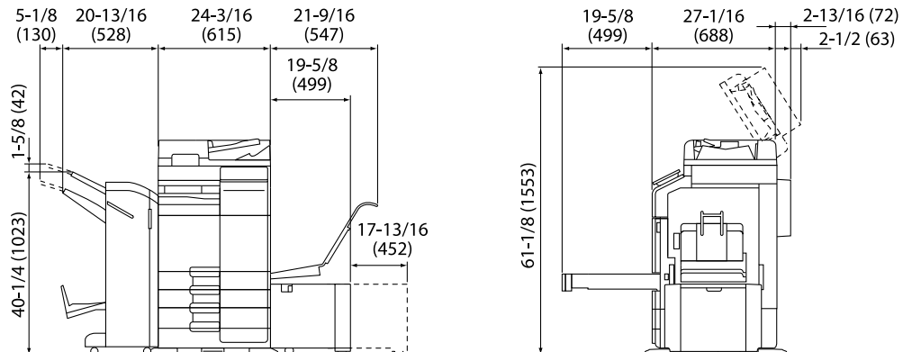
Βασική μονάδα + DF-714 + FS-539 SD + PC-216 + LU-302 + MK-730 + CU-102 Μονάδα: ίντσα (mm)
